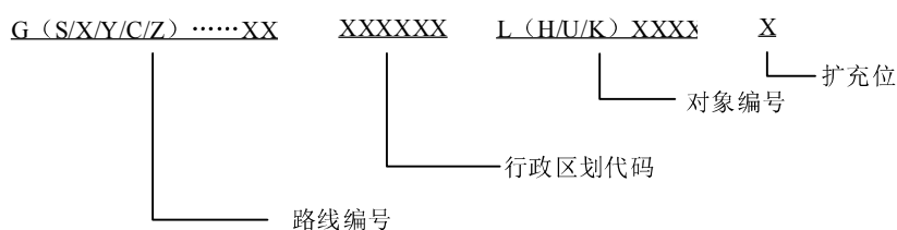
图 4-1 代码结构
